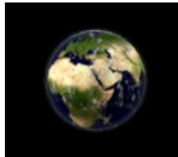
Terraform 1.0
